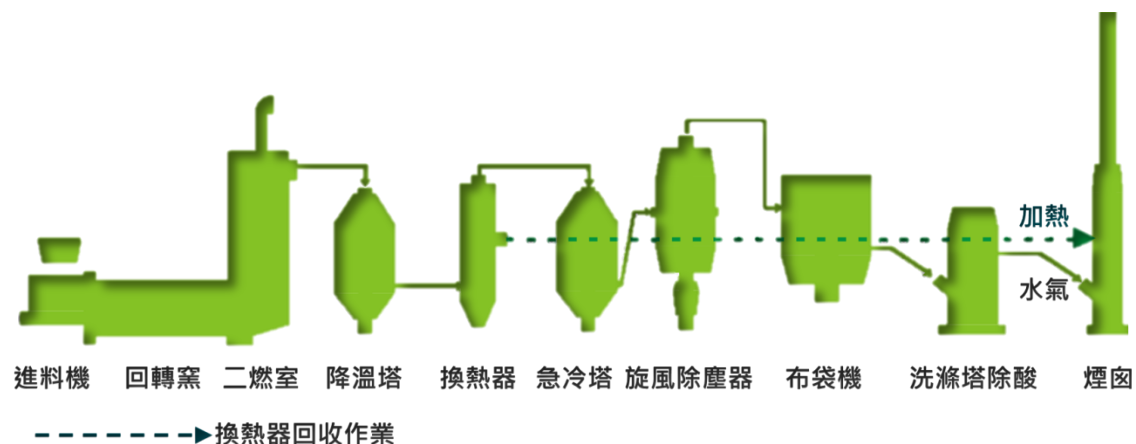
▲廢棄物焚化設備處理流程示意圖
